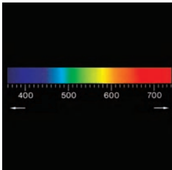
▲ تصویر ۴-۸ طول موج نورهای مختلف
